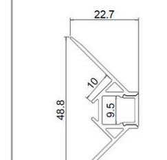
LEX/MID070 dimensions
