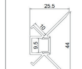
LEX/MID069 dimensions
