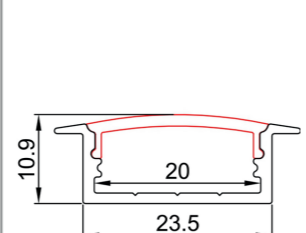
LEX/MID013 dimensions
