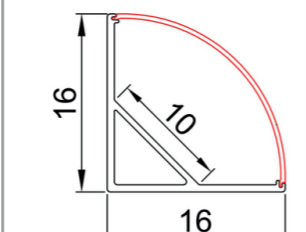
LEX/MID006 dimensions
