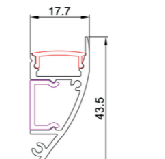
LEX/MID062 dimensions
