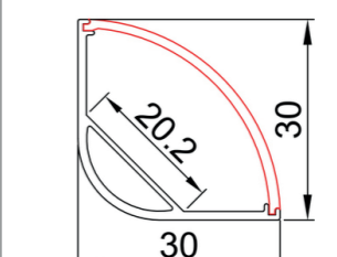
LEX/MID016-R dimensions
