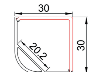
LEX/MID015-R dimensions
