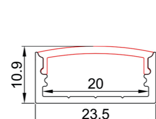
LEX/MID014 dimensions
