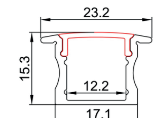
LEX/MID003-R dimensions
