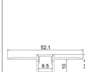
LEX/MID068 dimensions
