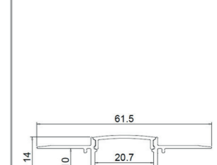
LEX/MID071 dimensions
