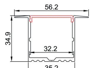
LEX/R/B dimensions
