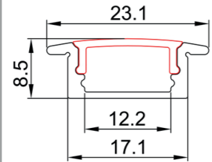
LEX/R/SLIM dimensions
