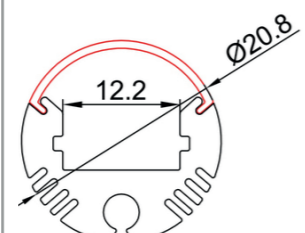
LEX/MID008 dimensions
