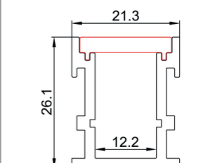
LEX/MID034 dimensions
