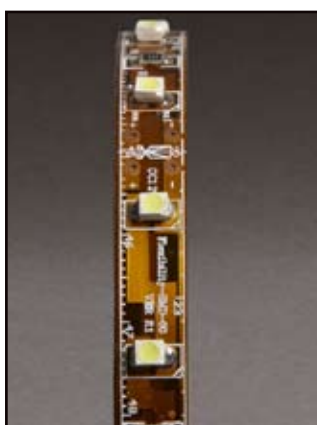
60 LEDs/m - 4.8W/m
