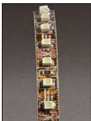
120LEDs/m - 9.6W/m
